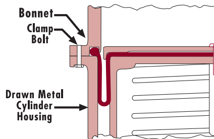
Fig. 30: Grooved Bonnet
