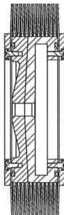
SECTION A-A
