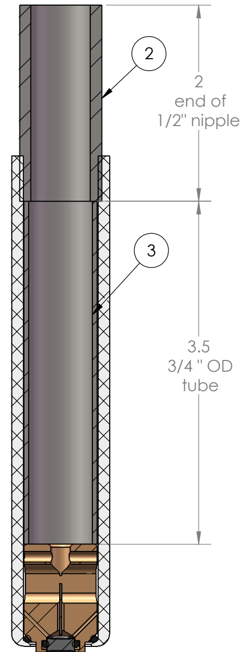
SECTION A-A SCALE 1 : 1
