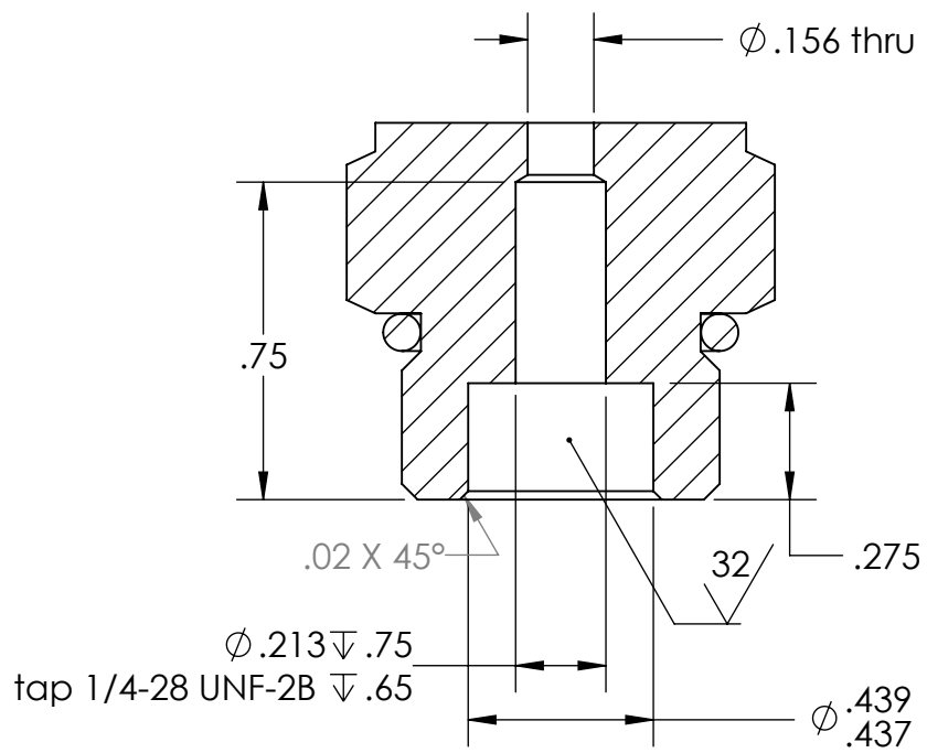
SECTION A-A
