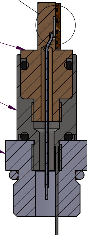
SECTION D-D SCALE 2 : 1
