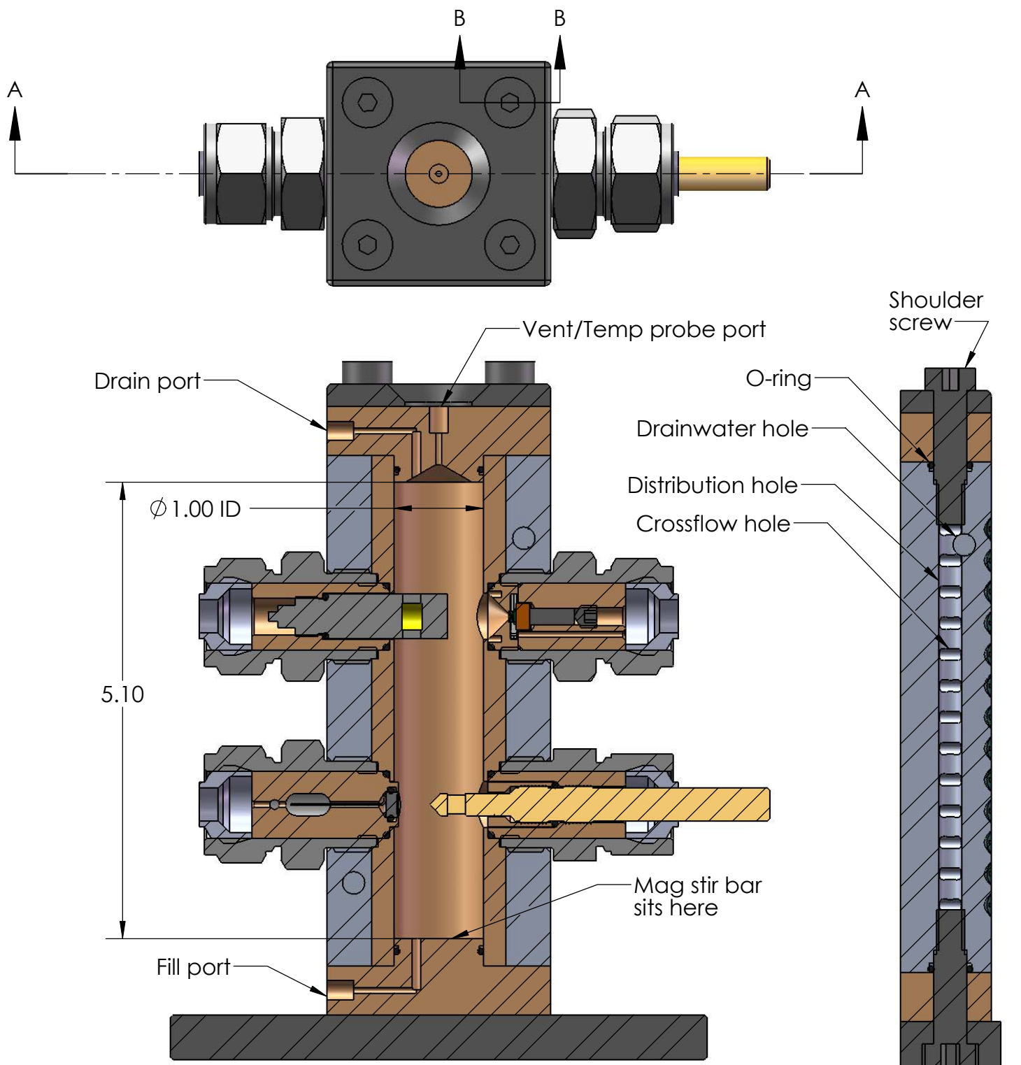
SECTION A-A SCALE 1 : 1.5
