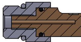
SECTION A-A SCALE 1 : 1
