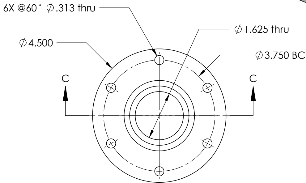
Al Mast Taper
