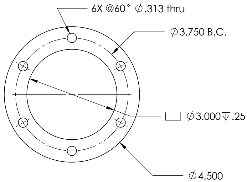
Al Frame ring
