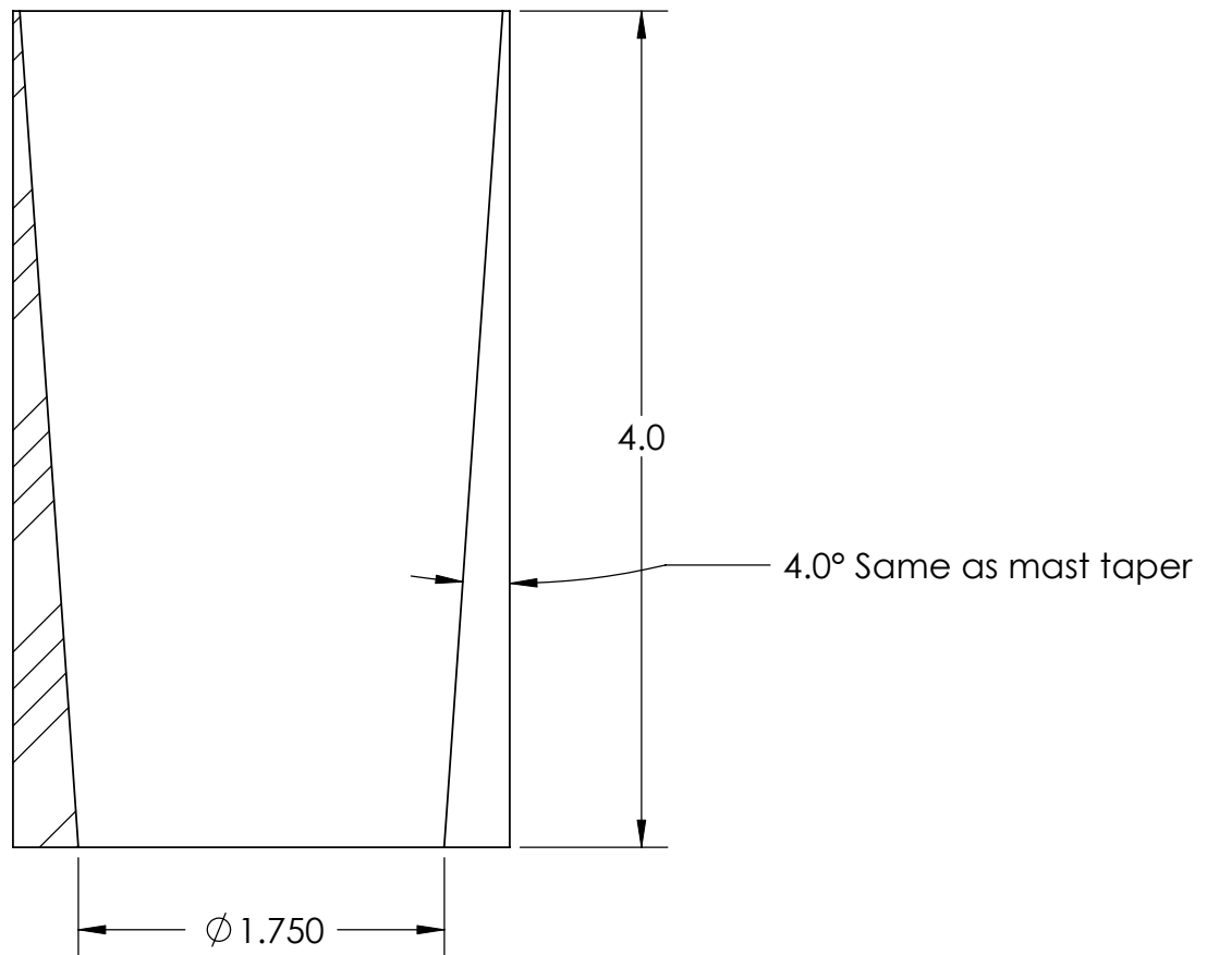
SECTION D-D SCALE 1 : 1
