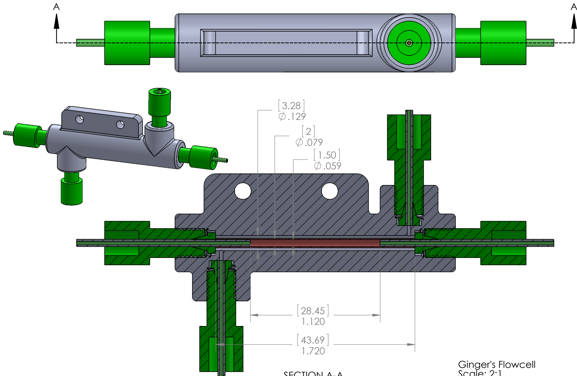
SECTION A-A SCALE 2 : 1
