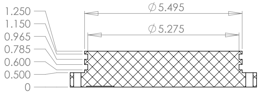
SECTION A-A SCALE 1 : 2
