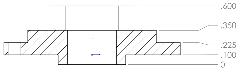
SECTION A-A SCALE 2 : 1
