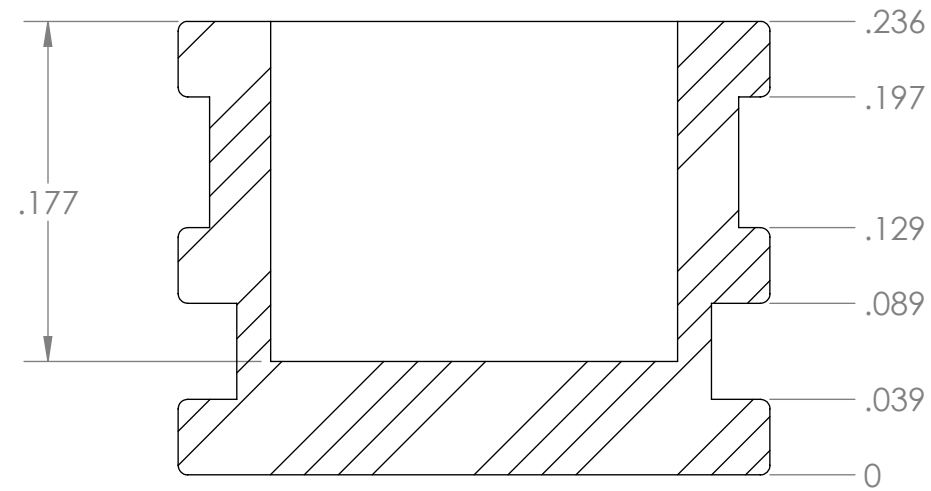
SECTION A-A SCALE 10 : 1
