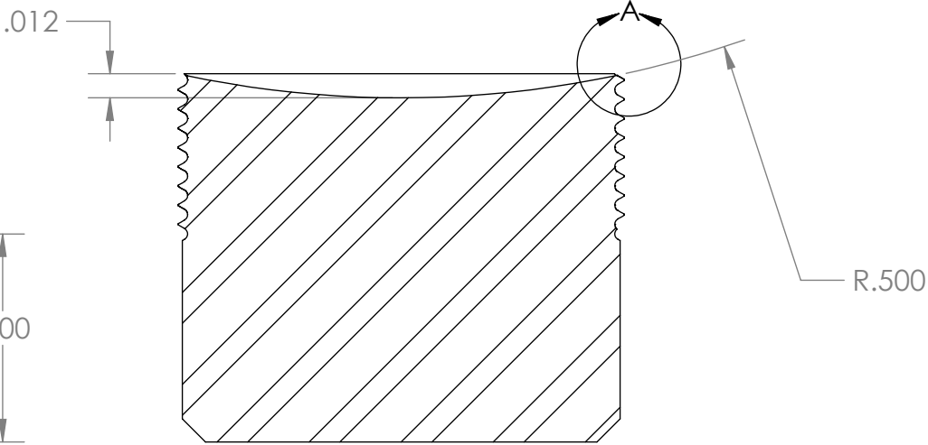
SECTION B-B SCALE 12 : 1
