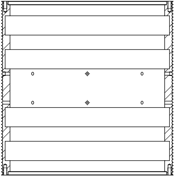
SECTION A-A SCALE 1 : 4
