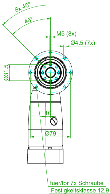
Ansicht von rechts / view from right
