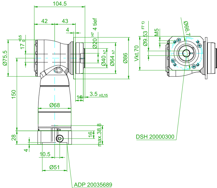
Ansicht von unten / view from bottom
