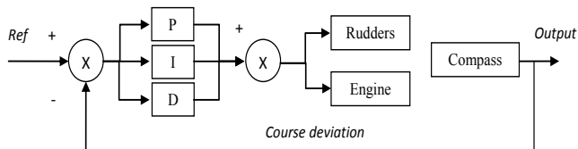
Fig. 1. PID controller.
