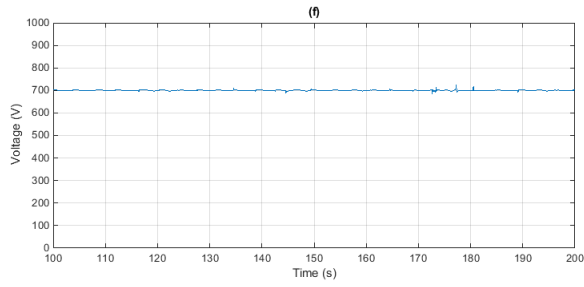
Fig. 15. DC bus voltage
