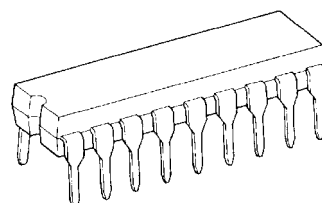
DIP18-P-300-2.54F
