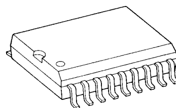
SOL18-P-300-1.27
