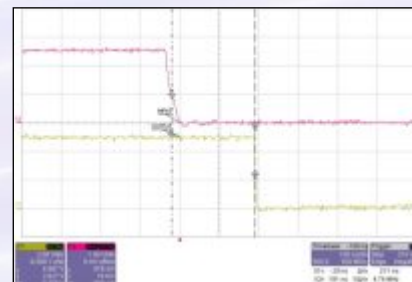
Falling Edge (100nSec/Div.)
