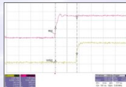
Rising Edge (100nSec/Div.)
