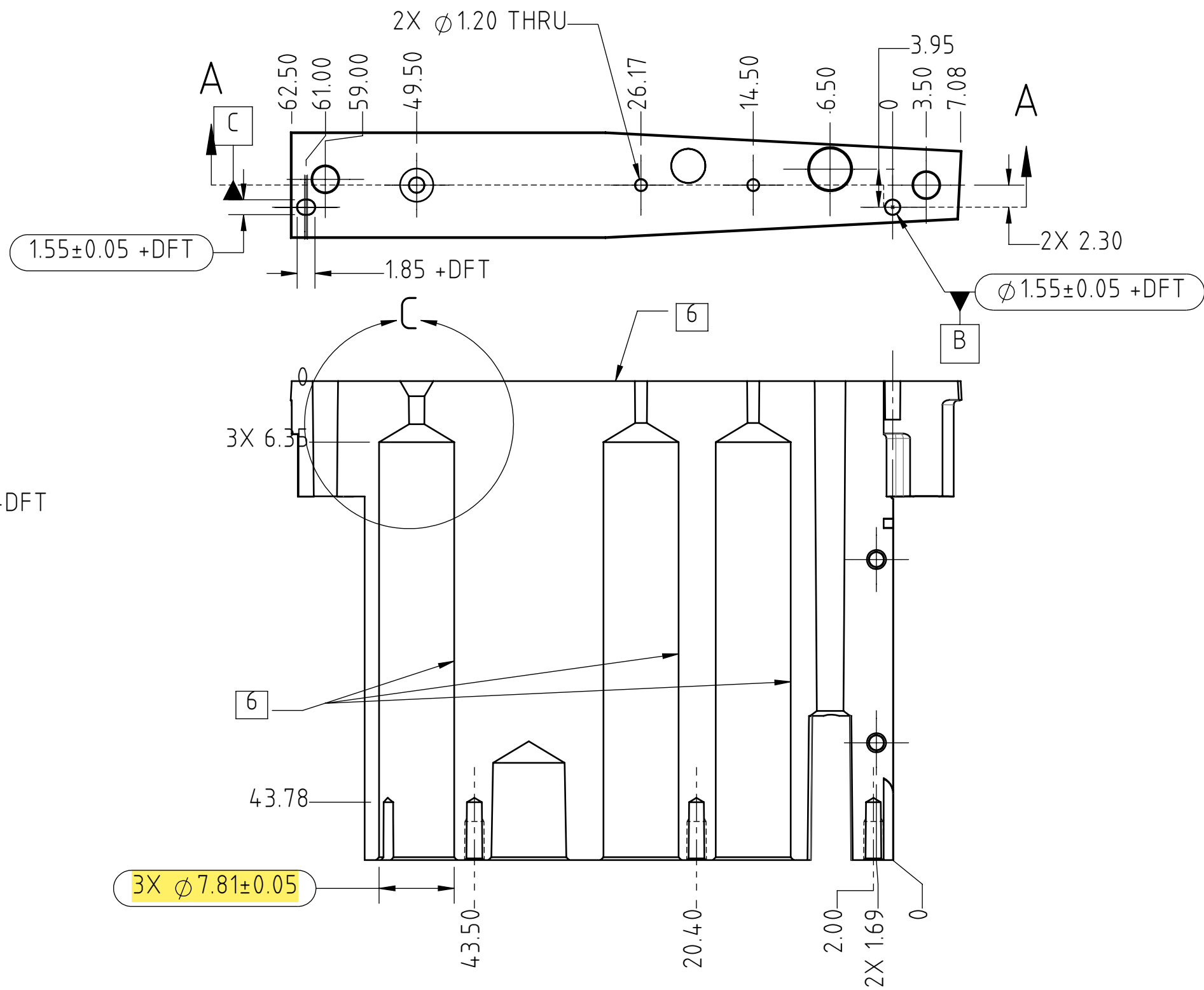
SECTION A-A
