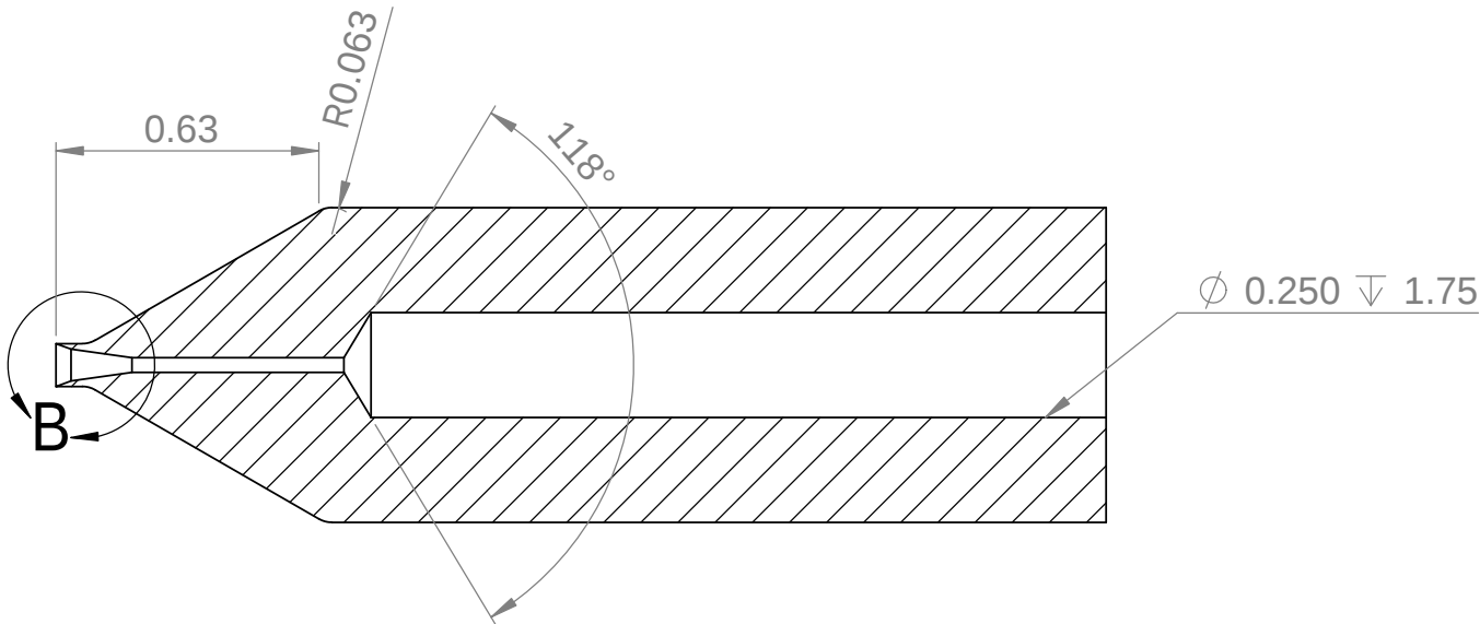
SECTION A-A SCALE 2 : 1
