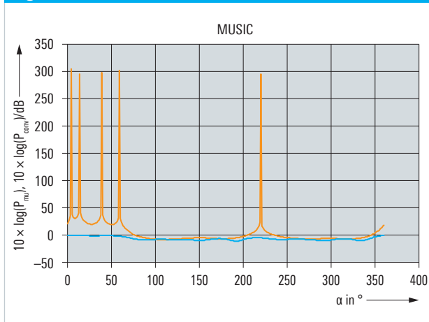
Fig. 28: DF function
