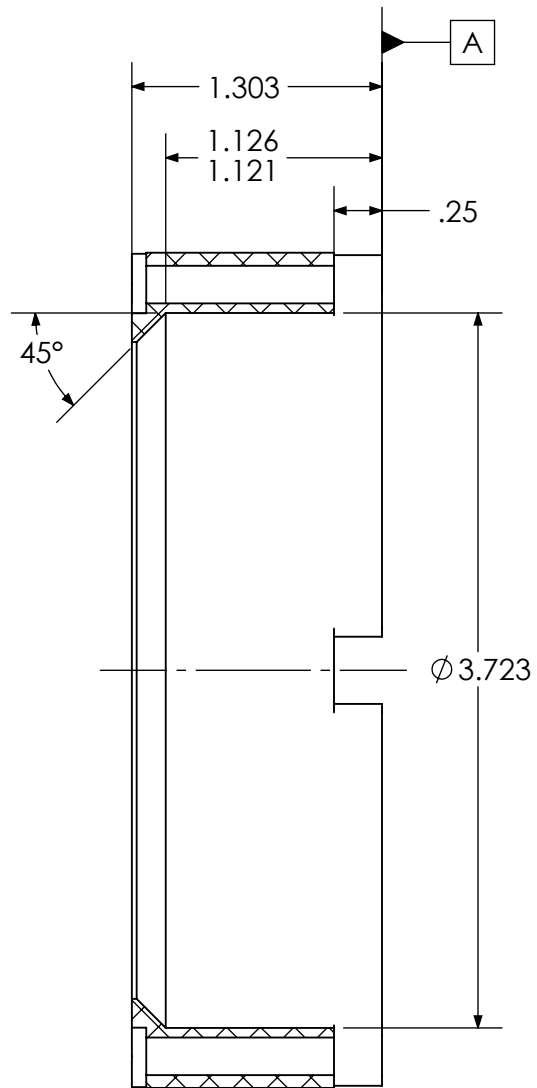
SECTION A-A
