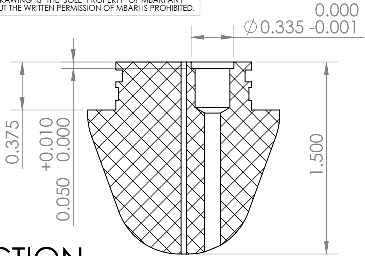
SECTION A-A SCALE 2 : 1.5
