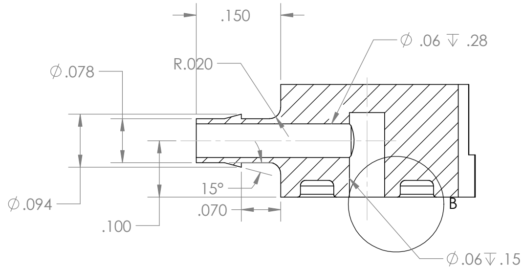
SECTION A-A SCALE 6 : 1
