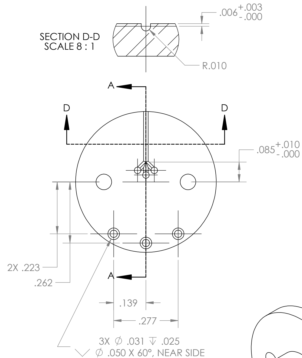
SECTION A-A
