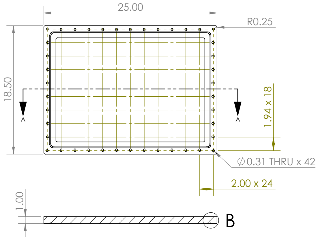
SECTION A-A SCALE 1 : 8
